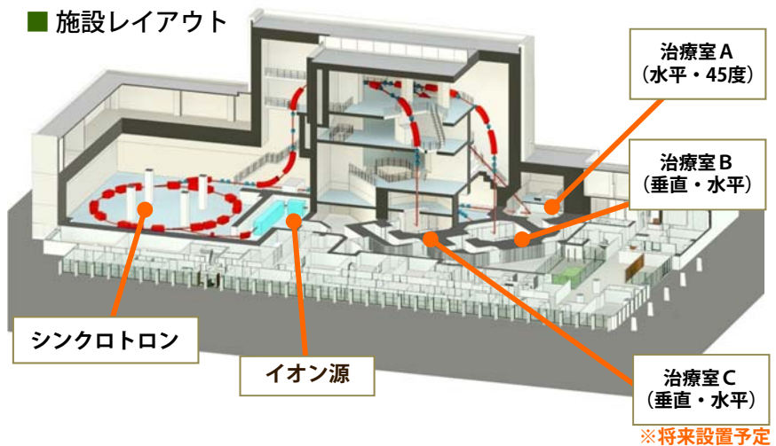
重粒子線を垂直、斜め45度から照射するラインは、円周部分を出た後、建物の3階に引き上げられる。
